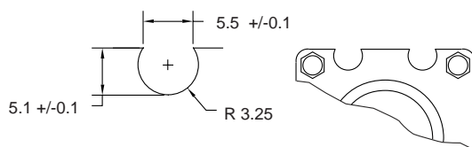
GROOVE DIMENSIONS
